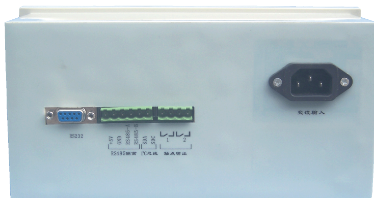
图 2 FYDXJ-2000-A 智能电参数巡检系统后面板图
