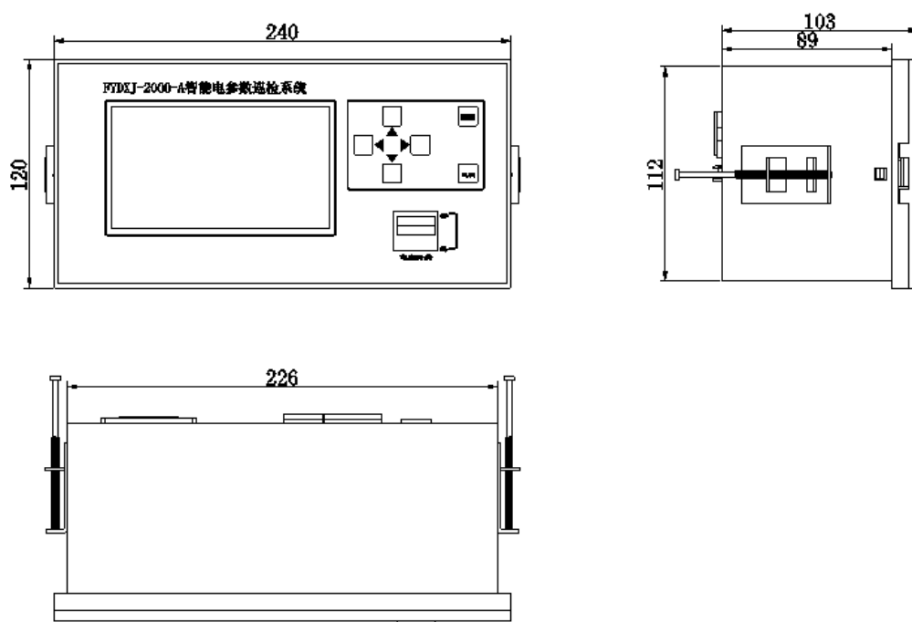
图 3 FYDXJ-2000-A 智能电参数巡检系统外形尺寸图
